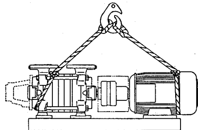
Abb. 2.1d Pumpen der Baureihe Z
