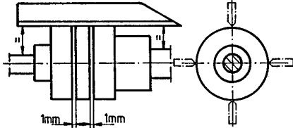
Abb. 4.1a Ausrichtung der Kupplung
