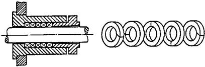
Abb. 6.2.3.3a Stopfbuchspackung
